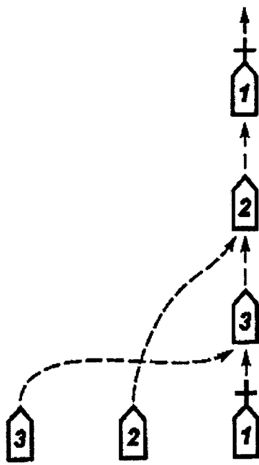
Рис. 44. Перестроение взвода из линии машин в колонну
