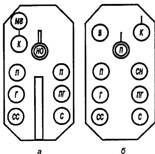
Рис. 40. Размещение личного состава: а - в боевой машине пехоты; б - в бронетранспортере
