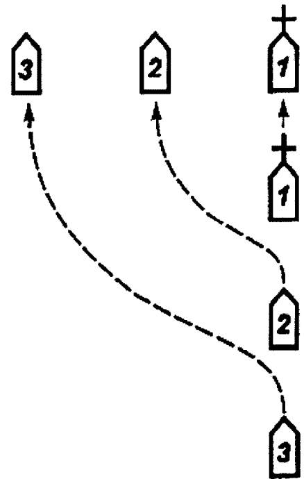
Рис. 45. Перестроение взвода из колонны в линию машин
