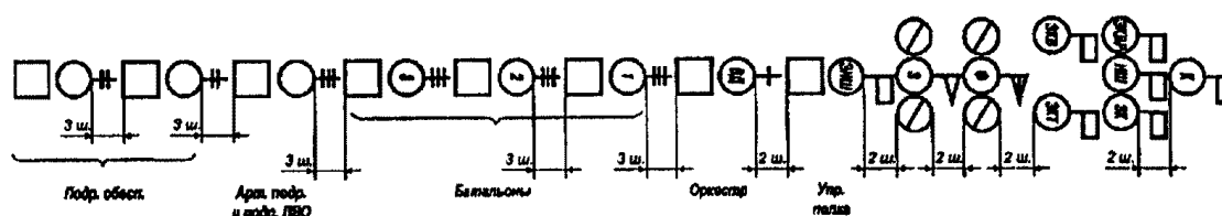
Рис. 34. Походный строй полка - колонна
